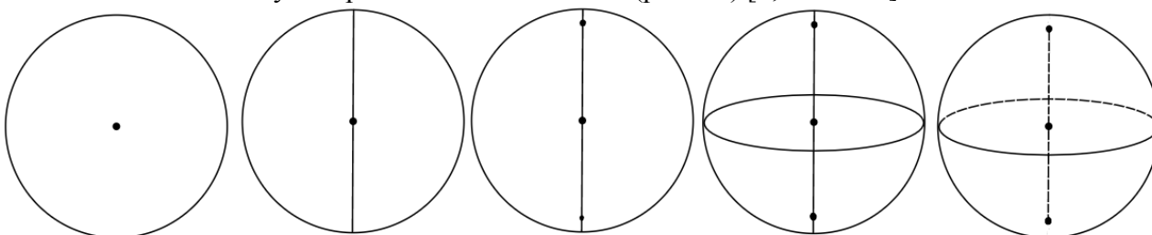
Рис. 13. Построение шара
