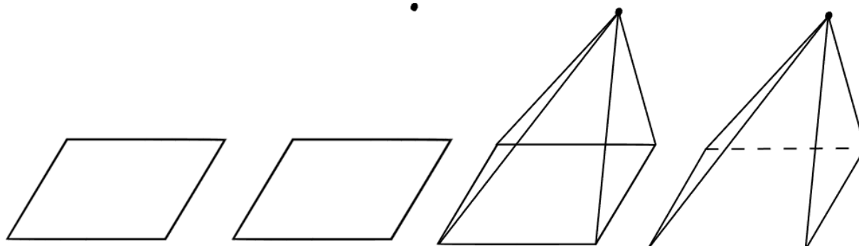
Рис. 10. Построение пирамиды
