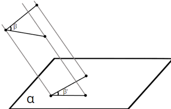
Рис. 3. Изображение угла
