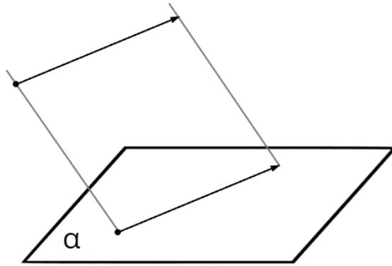
Рис. 1. Изображение луча
