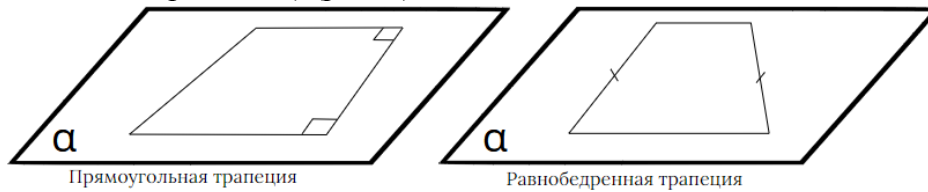
Рис. 6. Изображение трапеции
