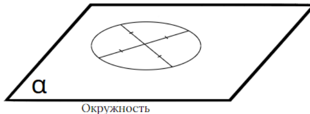
Рис. 8. Изображение окружности
