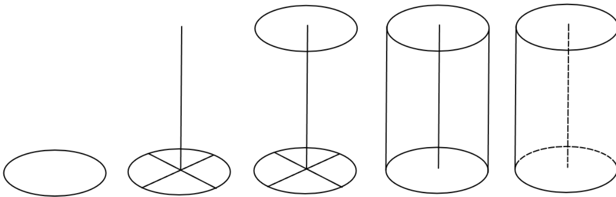
Рис. 11. Построение цилиндра
