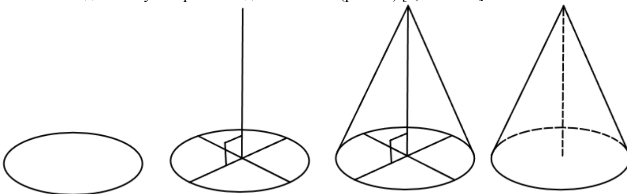
Рис. 12. Построение конуса
