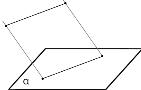
Рис. 2. Изображение отрезка
